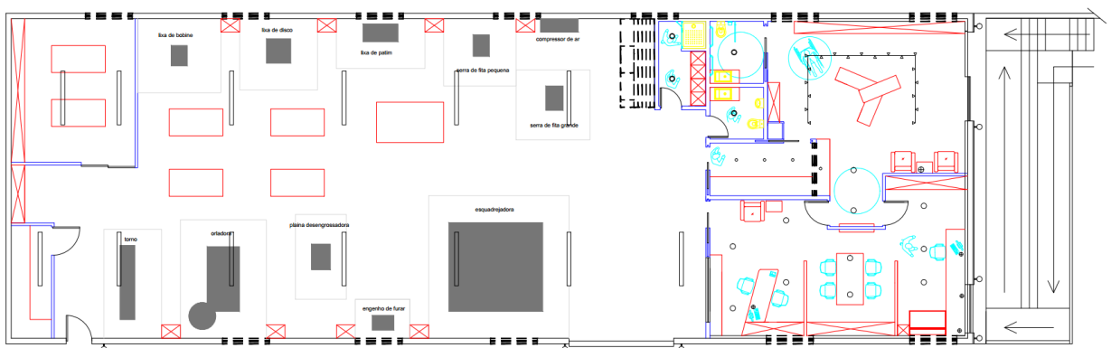
Ilustração 26: Planta de Equipamento com Iluminação
