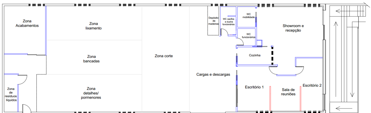
Figura 25: Planta zoneamento
