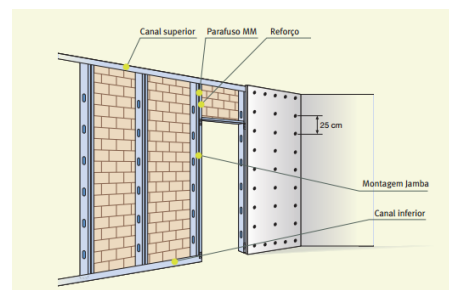
Ilustração 16: Sistema de paredes em pladur para conforto sonoro e térmico
