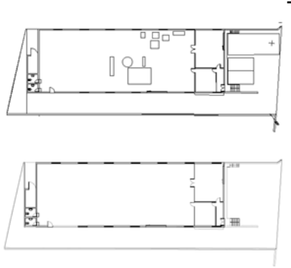
Ilustração 28: Planta original com disposição actual da maquinaria
