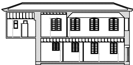
Fig. 3 Corte - Existente
