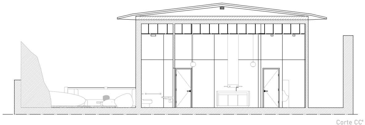
Figura 93 - Corte CC' Fonte: Patrícia Mateus
