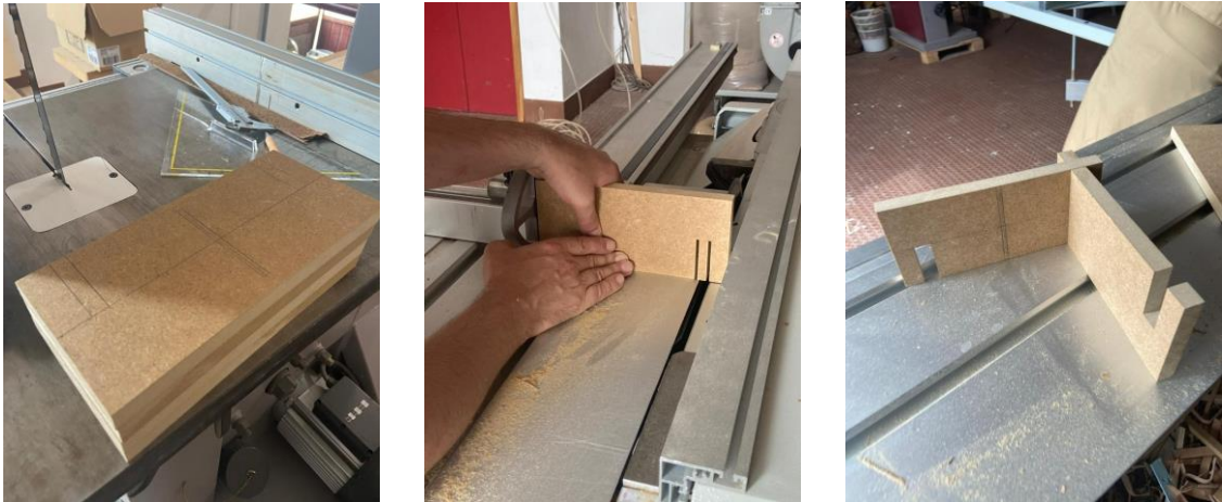
Figuras 79,80,81 – Imagens do Processo de Execução em Oficina, Marcação das peças, Cortes e Execução dos encaixes, Fonte: Autor
