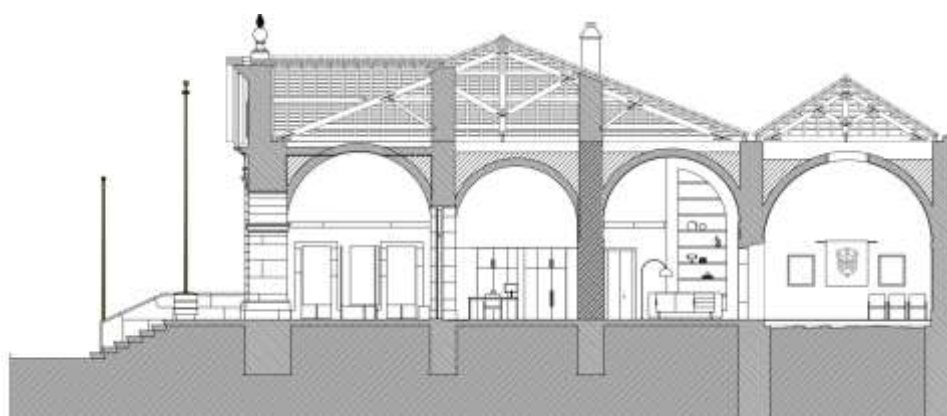
Figura 73. Corte CC'
