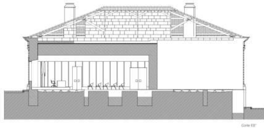
Figura 75. Corte EE'
