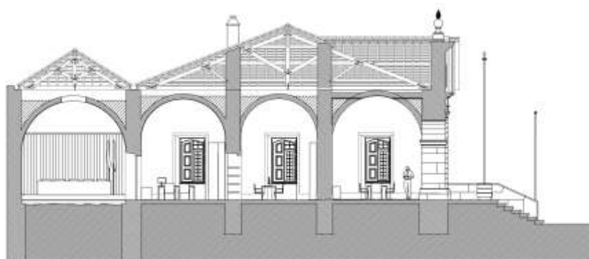
Figura 71. Corte AA'
