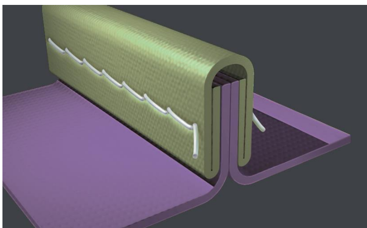
Figura 51 – Ilustração do tipo de costuras utilizadas nos fatos de banho de alta competição
