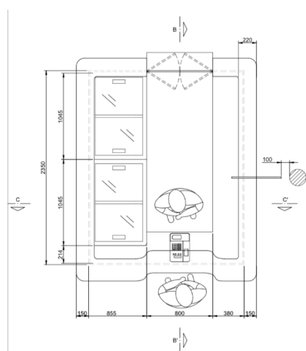
Figura 84 – Planta do equipamento. Fonte: Catarina Fernandes (2023)
