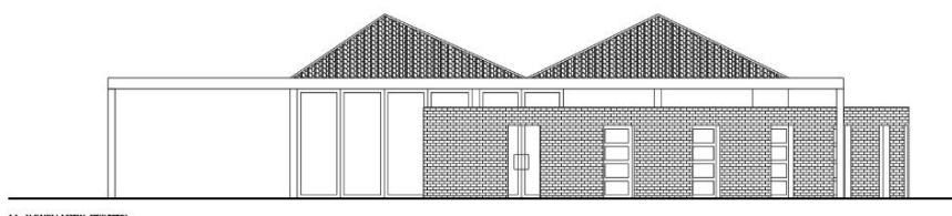
Figura 11 - Alçado lateral direito. Fonte: Paulo Amorim Arq. (2022)
