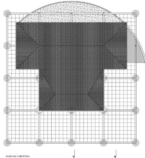
Figura 7 - Planta de Cobertura. Fonte: Paulo Amorim Arq. (2022)
