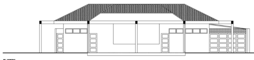
Figura 13 - Corte 02. Fonte: Paulo Amorim Arq. (2022)
