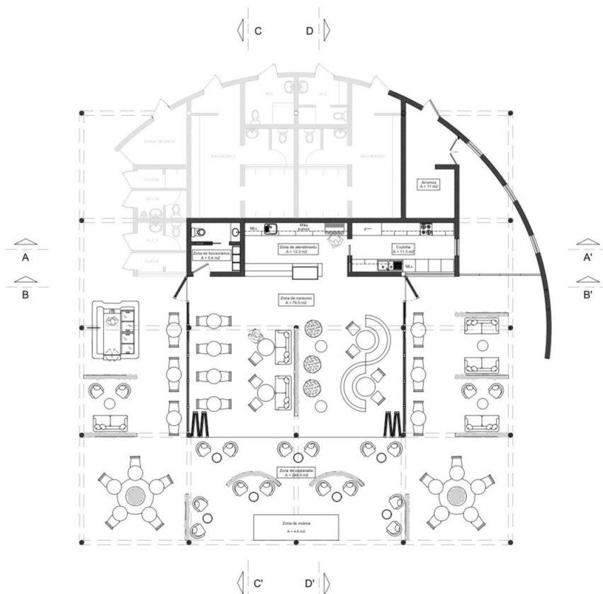
Figura 67 – Planta de Apresentação. Fonte: Catarina Fernandes (2023)
