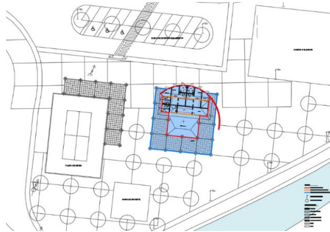
Figura 5 - Planta de Implantação. Fonte: Paulo Amorim Arq. (2022)
