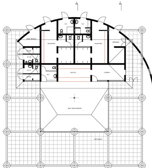
Figura 6 - Planta. Fonte: Paulo Amorim Arq. (2022)
