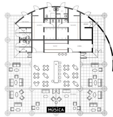
Figura 63 – Terceiro esboço. Fonte: Catarina Fernandes (2023)
