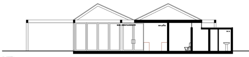
Figura 12 - Corte 01. Fonte: Paulo Amorim Arq. (2022)
