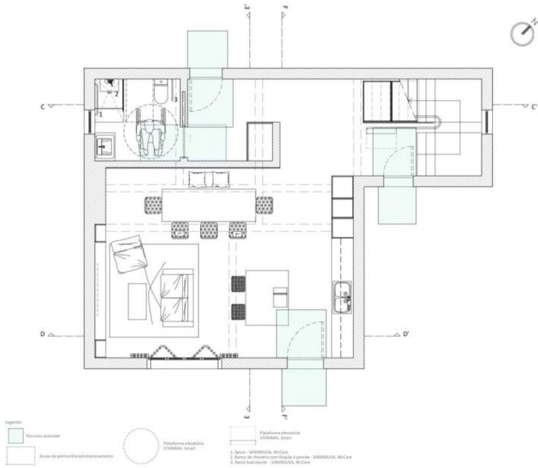
Figura 76 - Planta de Acessibilidades, Piso 0. Fonte: Autor
