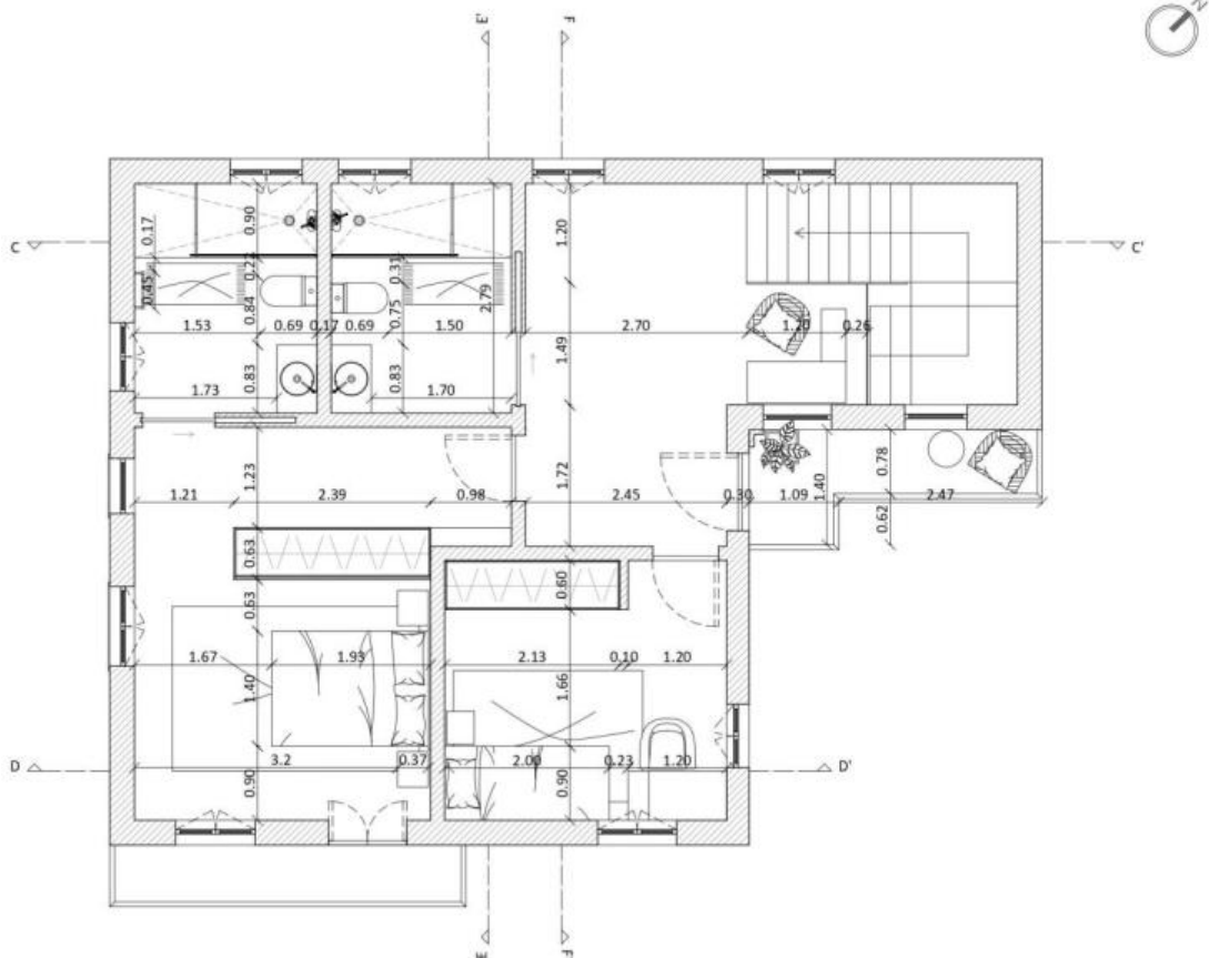
Figura 67 - Planta de Equipamento e Mobiliário cotada, Piso 1. Fonte: Autor
