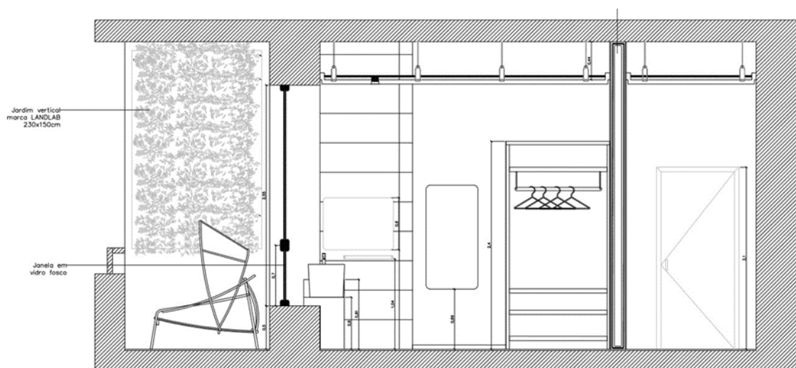
Figura 52: Pormenor Casa de Banho Quarto - Corte C - Escala 1:20
