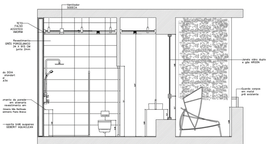
Figura 51: Pormenor Casa de Banho Quarto - Corte B - Escala 1:20
