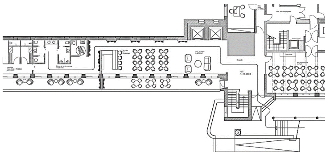
Figura 42: Planta de proposta - pormenor área de circulação piso 0
