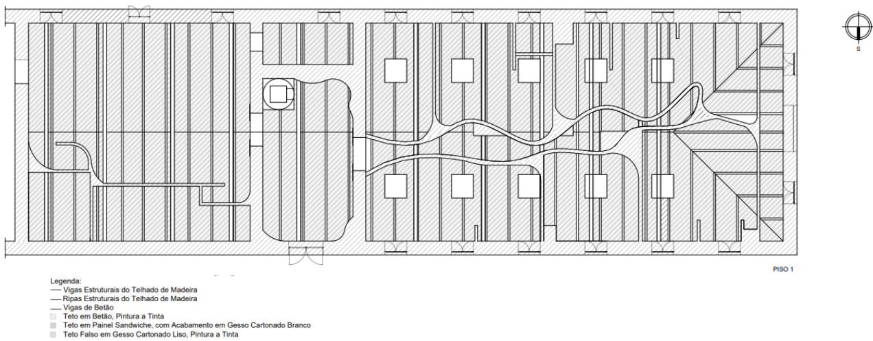
Figura 66 I - Planta de Tetos, Piso 1, Alojamento Olive
