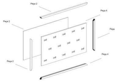
Figura 19- Axonometria e axonometria explodida da moldura. Fonte: Mafalda Coelho.
