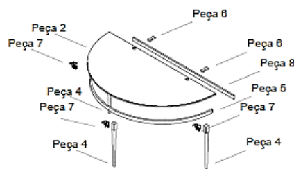
Figura 22- Axonometria e axonometria explodida do balcão. Fonte: Mafalda Coelho.
