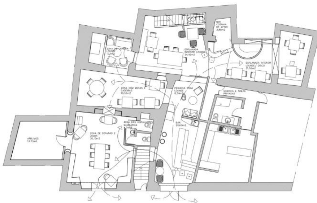
Figura 3-Planta de zonamentos e circulação do existente
