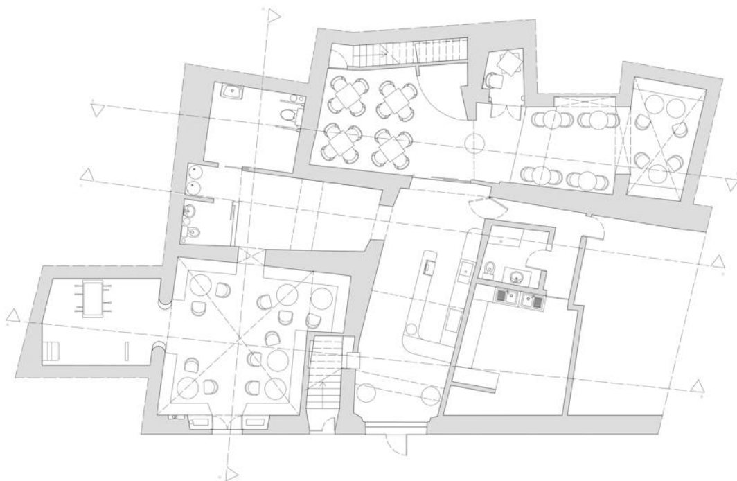
Figura 4-Proposta Final, Planta de Apresentação
