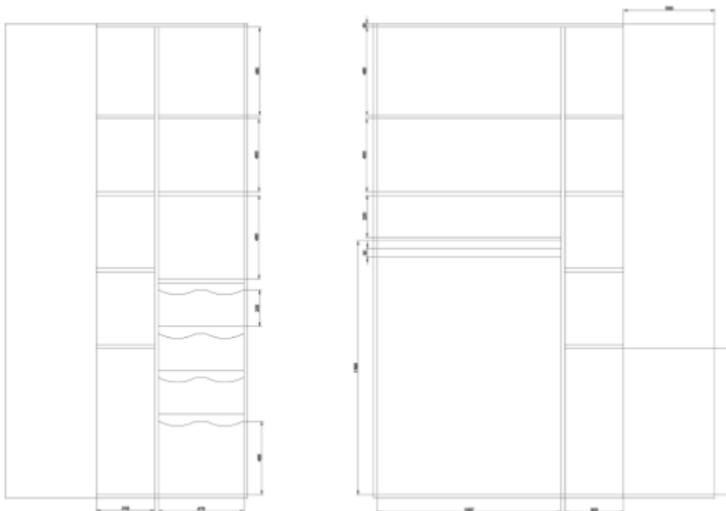
Figura 13- Desenho técnico do interior do armário ( Fonte : AutoCAD )
