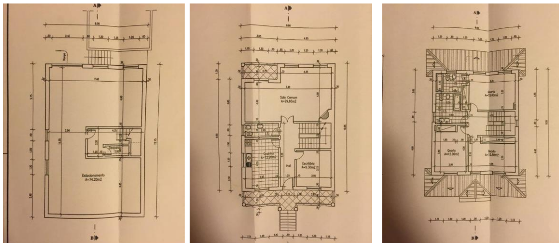
Figura 3- Planta Rés-do-Chão / Planta piso 1 / Planta piso 2
