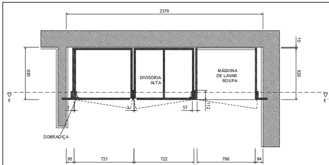
Figura 101: Parcela de desenho técnico de móvel lavandaria, André Bastos, 25\05\2023
