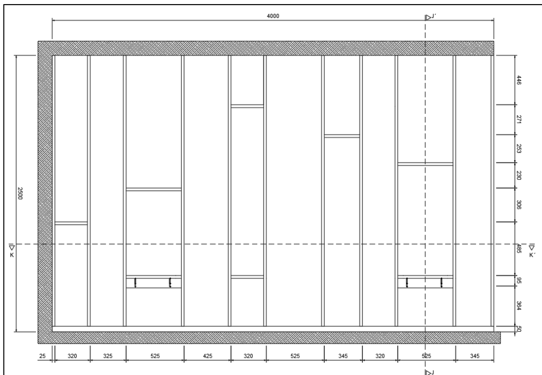
Figura 105: Parcela de desenho técnico de ripado quarto, André Bastos, 25\05\2023
