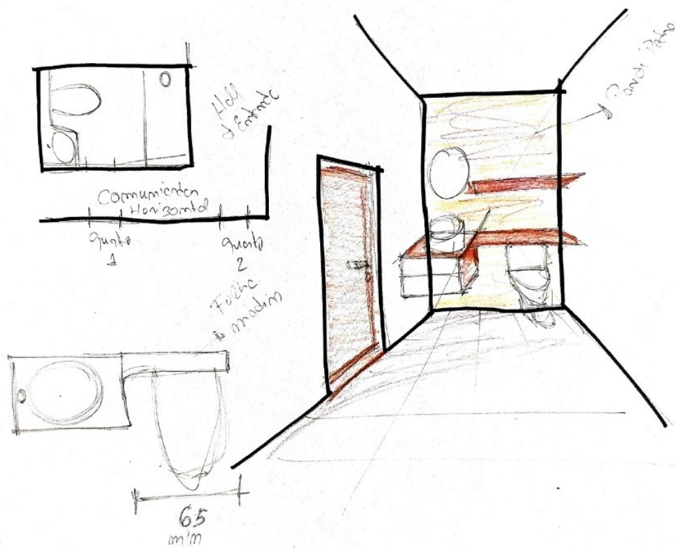
Figura 82: Instalação sanitária, móveis e vistas, desenho à mão levantada, André Bastos, 27\01\2023
