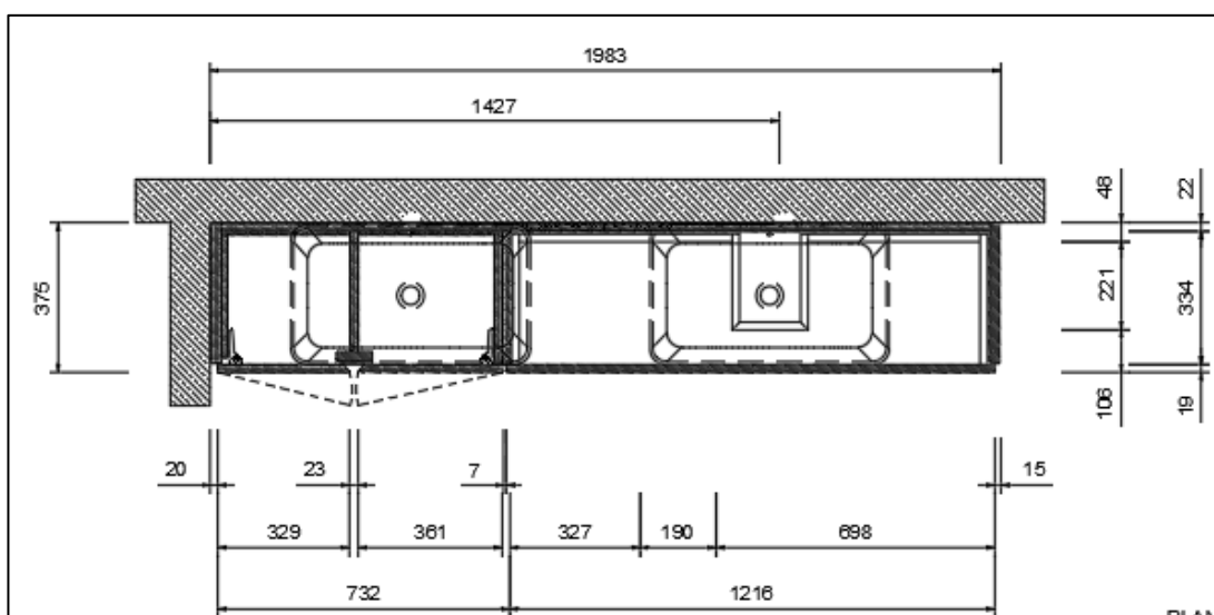
Figura 103: Parcela de desenho técnico de móvel instalação sanitária, André Bastos, 25\05\2023
