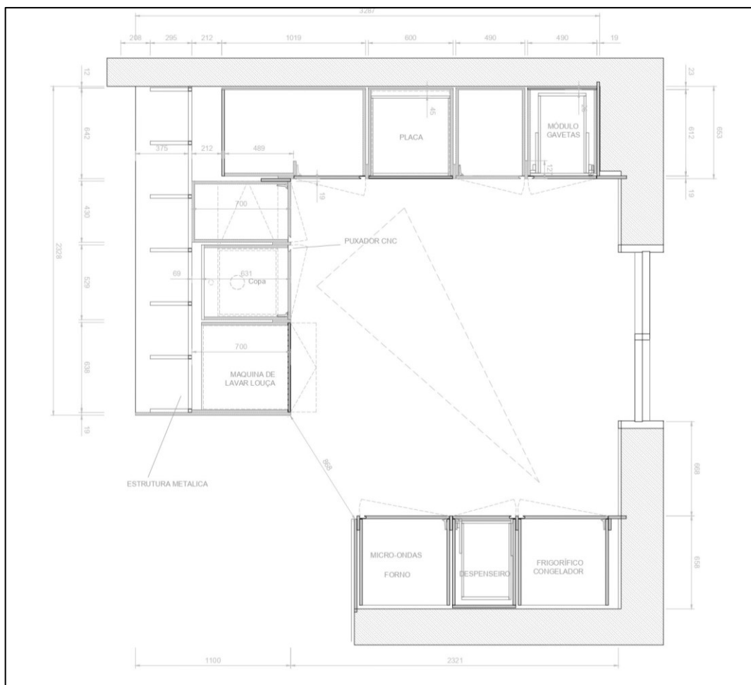
Figura 99: Parcela de desenho técnico de cozinha, André Bastos, 25\05\2023
