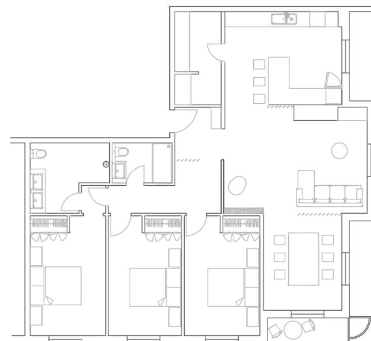
Figura 10: Esboço, planta 2d, autocad , André Bastos, 12\01\2023
