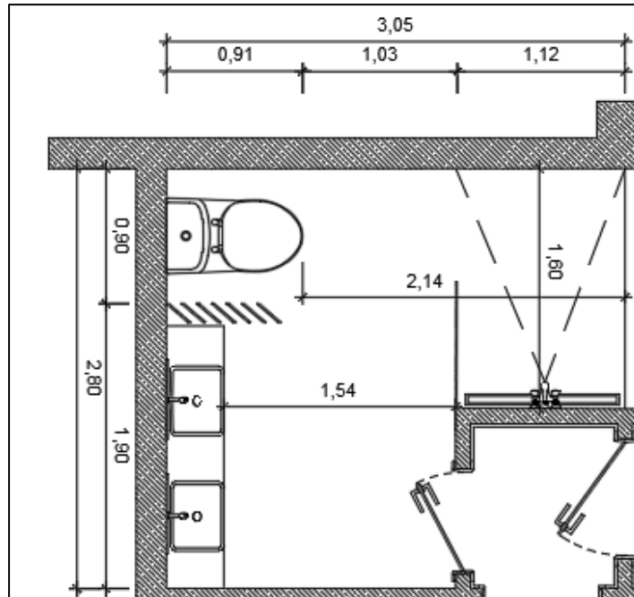
Figura 95: Parcela de desenho técnico de planta cotada, Instalação sanitária suite, André Bastos, 25\05\2023
