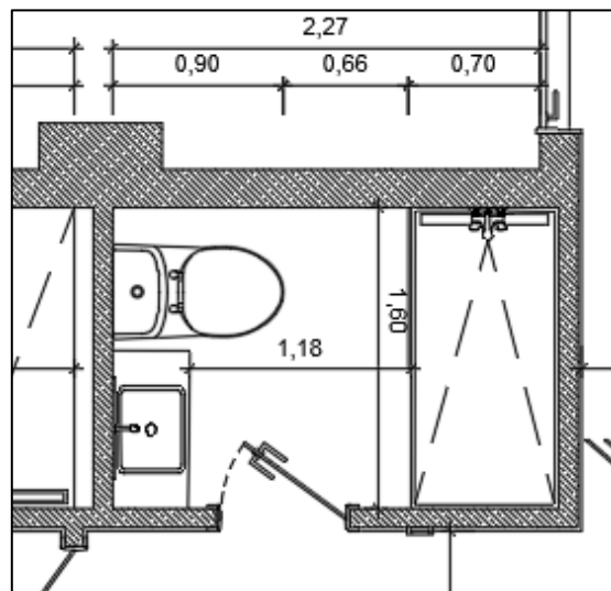
Figura 93: Parcela de desenho técnico de planta cotada, Instalação sanitária comum, André Bastos, 25\05\2023
