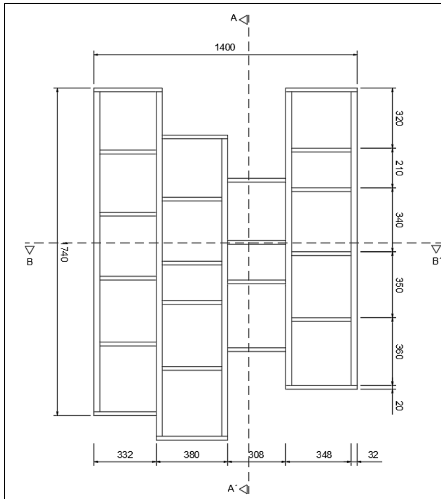
Figura 107: Parcela de desenho técnico móvel estante, André Bastos, 25\05\2023
