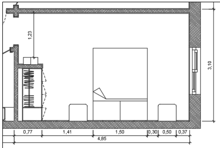
Figura 97: Parcela de desenho técnico da planta cotada, Quarto, André Bastos, 25\05\2023
