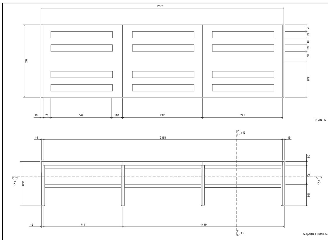
Figura 109: Parcela de desenho técnico de móvel sofá, André Bastos, 25\05\2023
