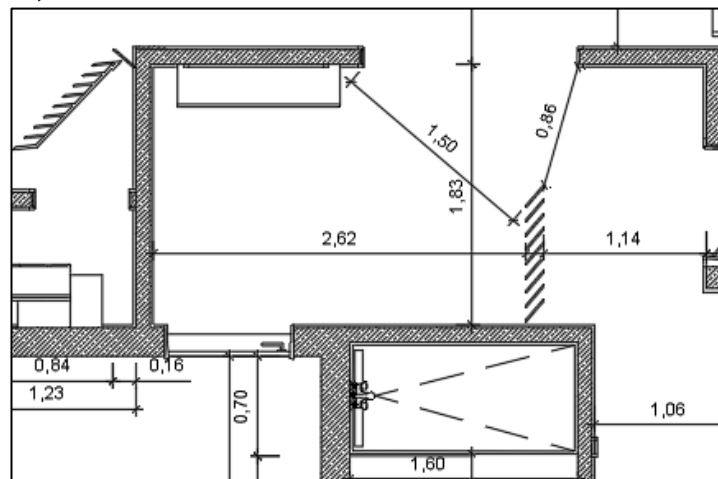
Figura 87: Parcela de desenho técnico, planta cotada, Hall de entrada, André Bastos, 25\05\2023
