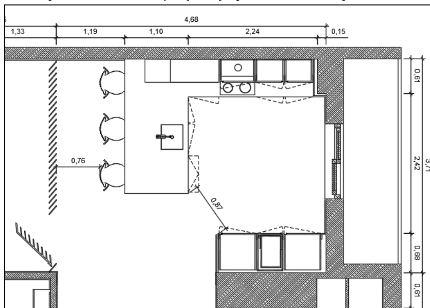
Figura 89: Parcela de desenho técnico de planta cotada, Cozinha, André Bastos, 25\05\2023
