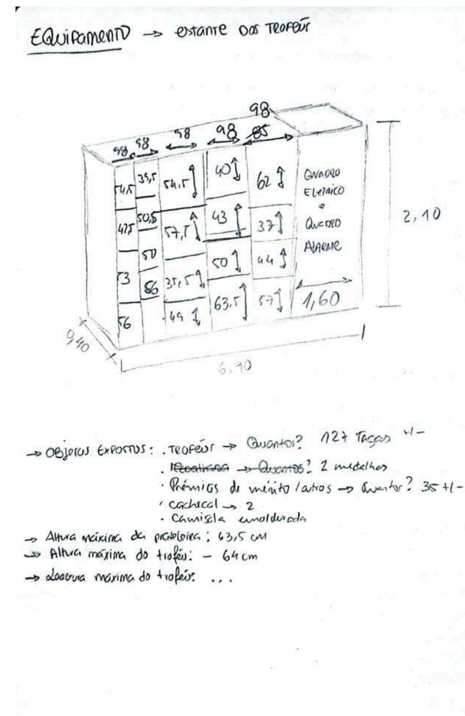
Figura 32- Levantamento do Equipamento
