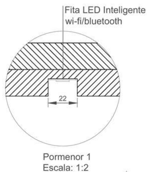
Figura 34- Pormenor da fita LED
