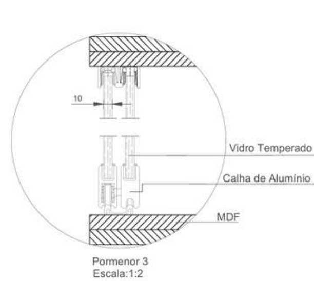
Figura 35- Pormenor das portas de correr
