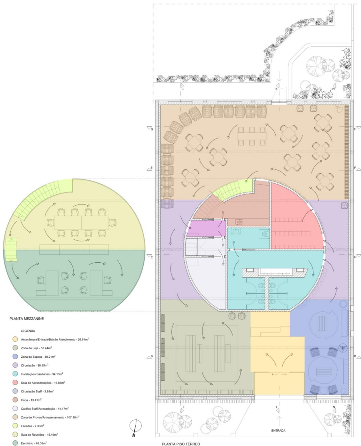
Figura 5 - Desenho Técnico - Planta de Circulação e Zoneamento. Fonte: (Autor)
