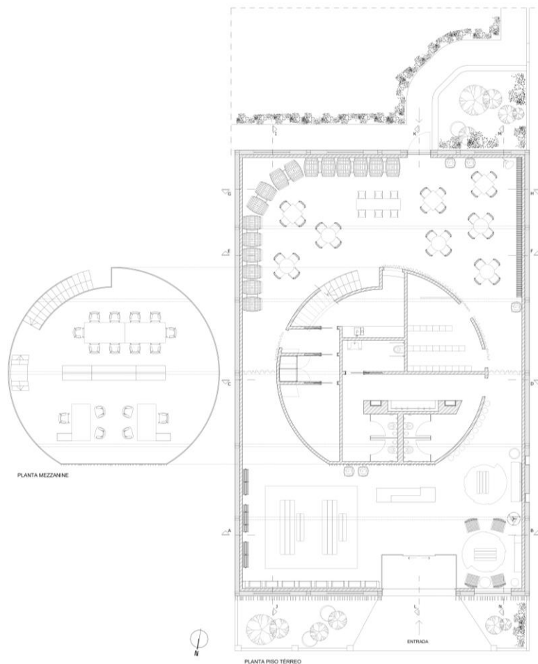
Figura 4 - Desenho Técnico - Planta de Apresentação. Fonte: (Autor)
