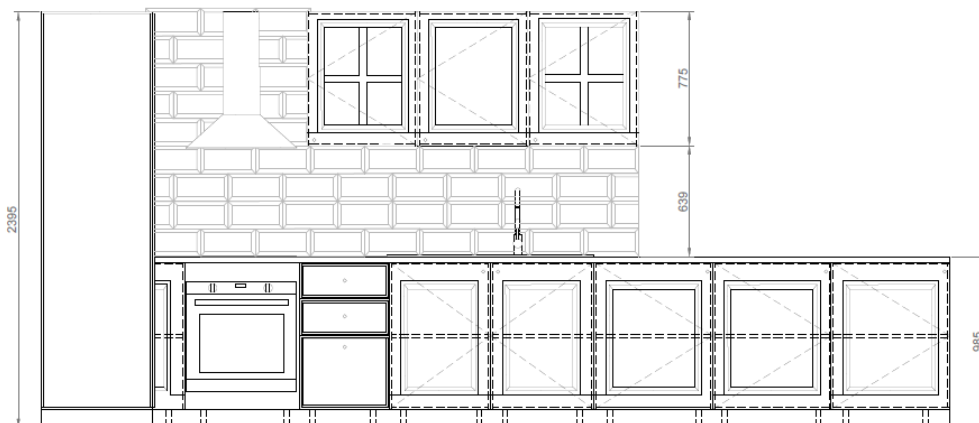
Figura 26 - Esquemático da cozinha.
