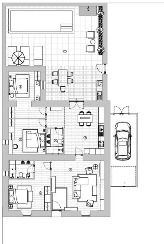
Figura 23- Planta de Proposta.
