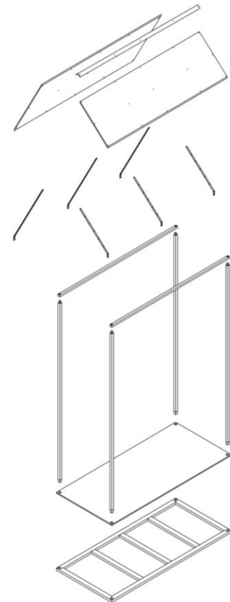
Figura 29- Axonometria
