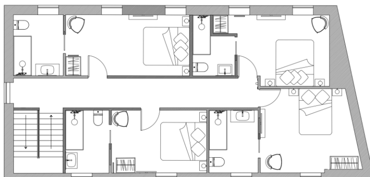
Figura 48 - Planta de estudo - Piso 1
