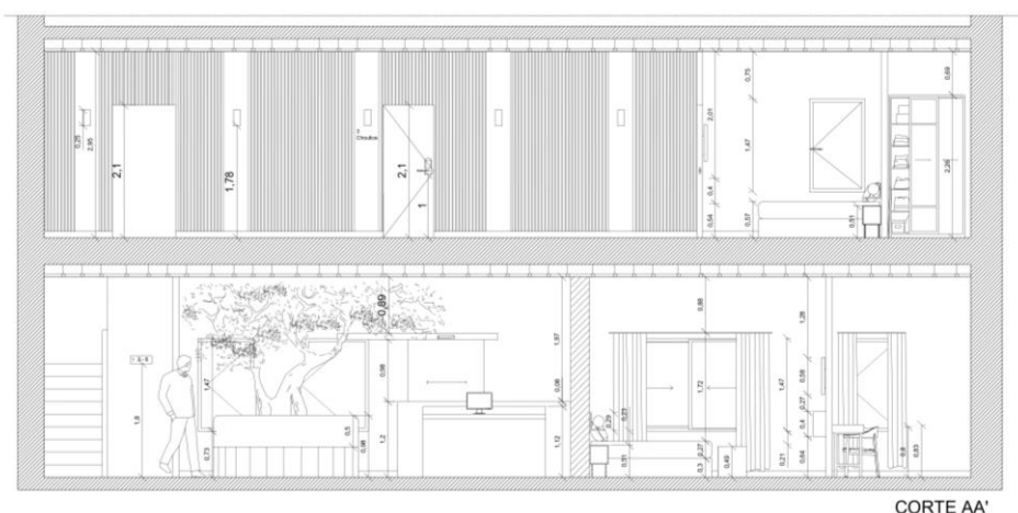
Figura 52 - Corte AA
