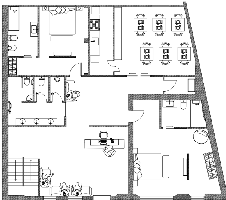
Figura 47 - Planta de Estudo - Piso 0
