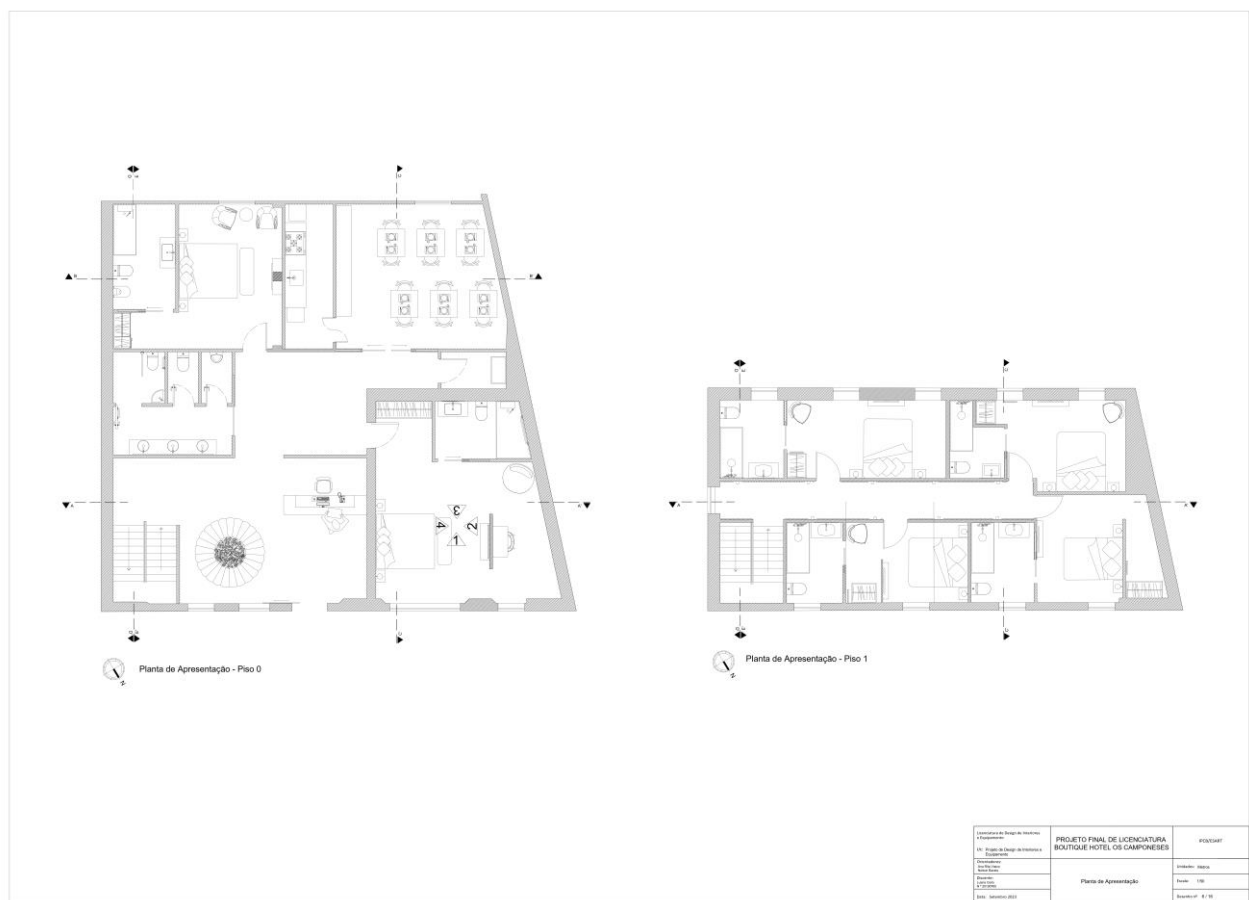
Figura 50 - Planta de Apresentação
