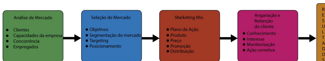
Figura 6 - Planeamento estratégico
