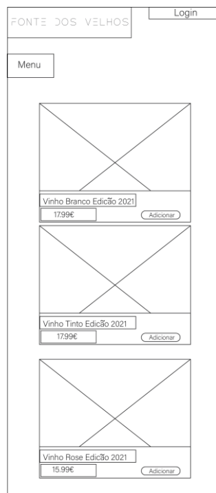
Figura 63 - Wireframe aplicação
