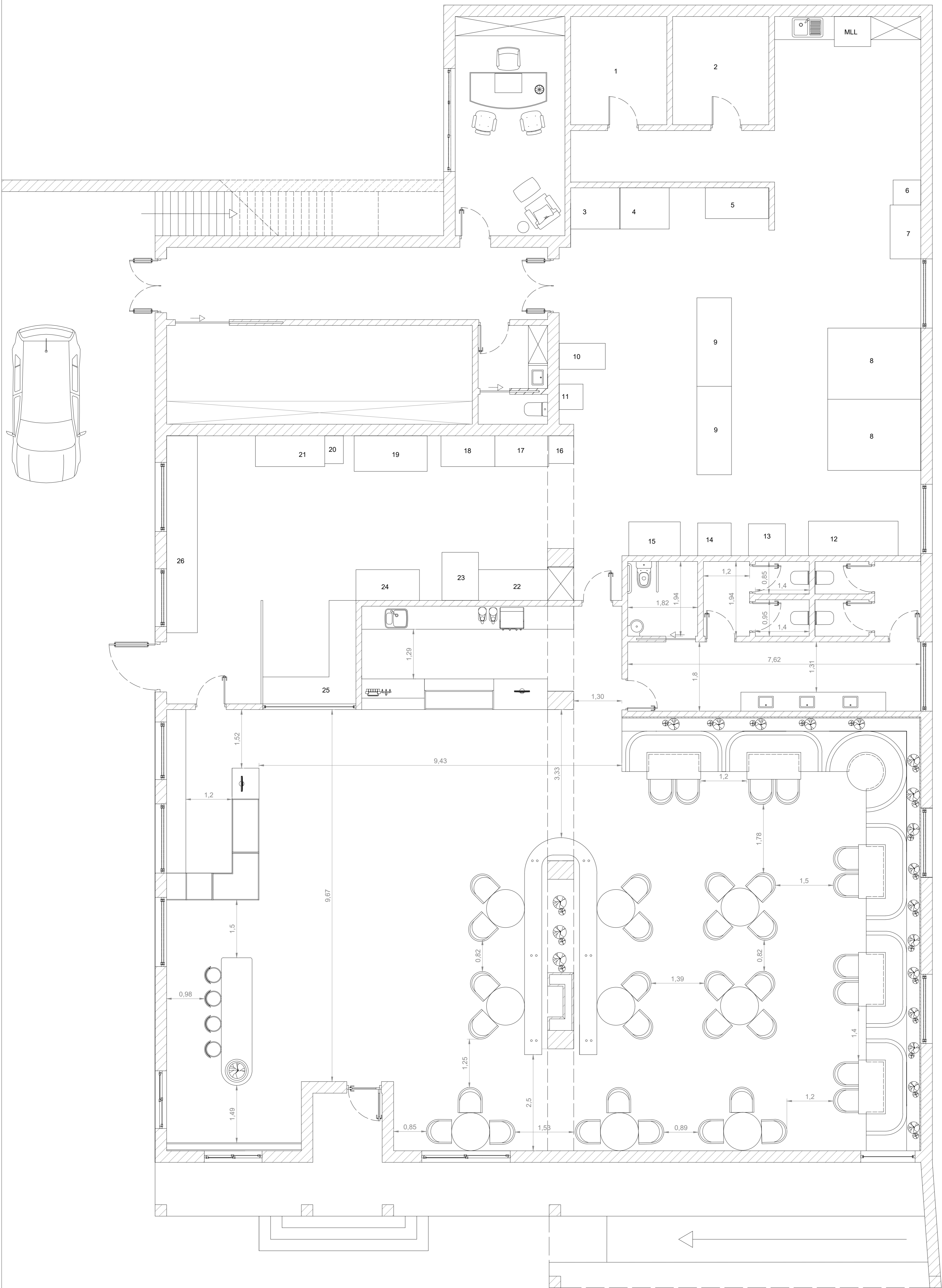
PLANTA DE APRESENTAÇÃO COTADA ESCALA 1/50
