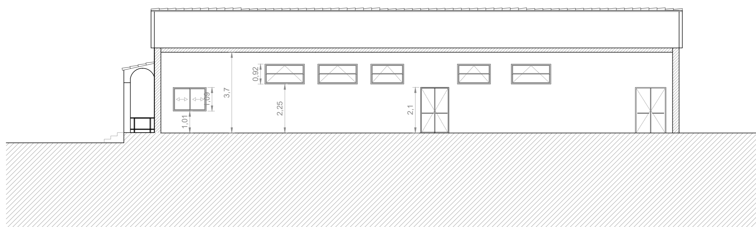
CORTE DD'
