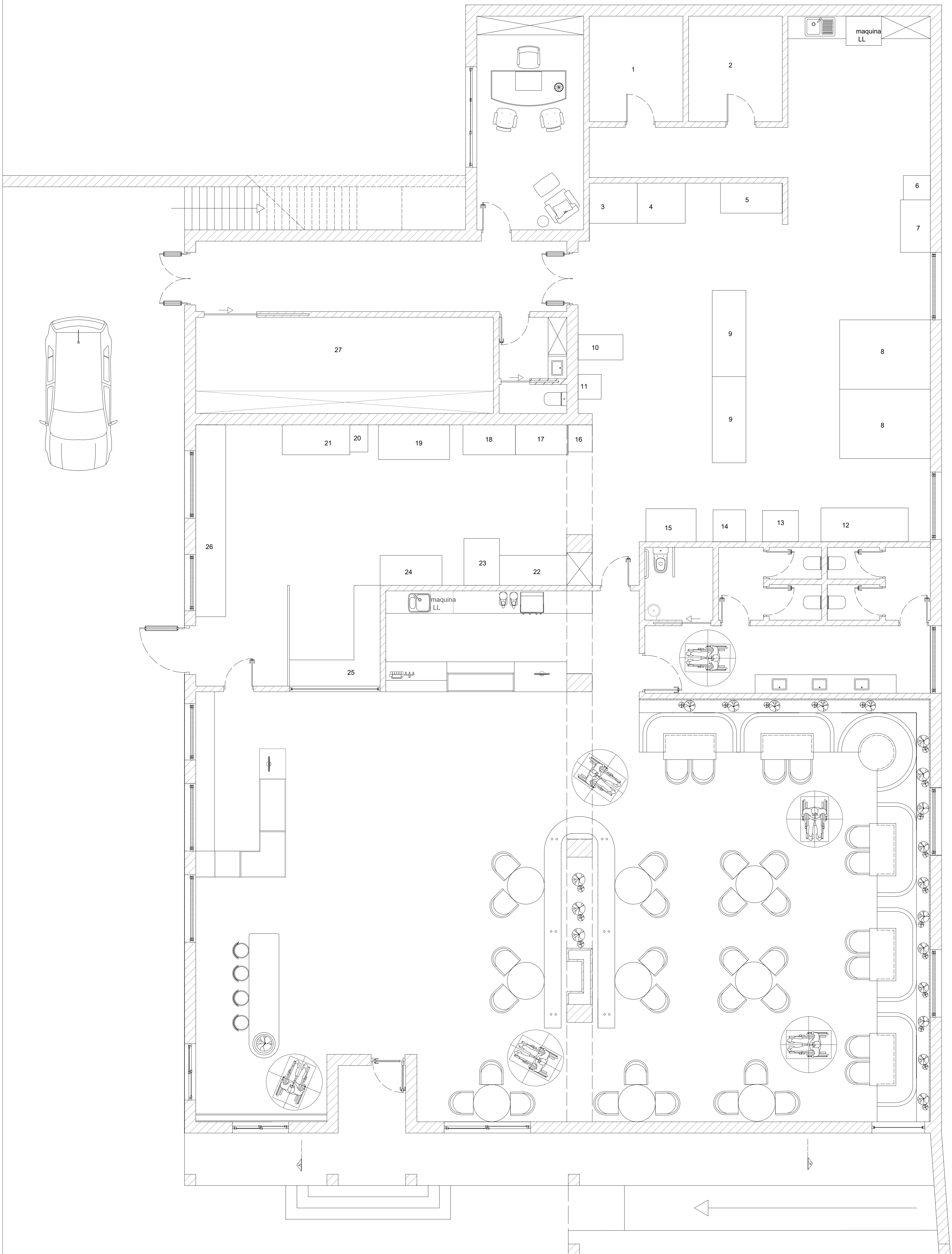
PLANTA DE ACESSIBILIDADES ESCALA 1/50
