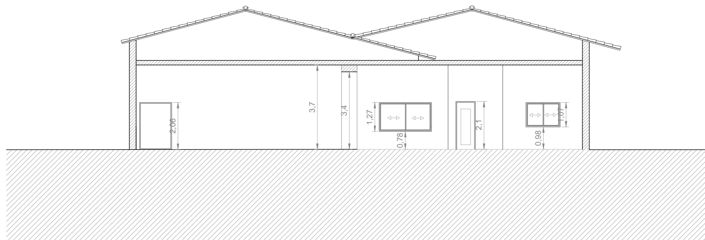
CORTE AA'
