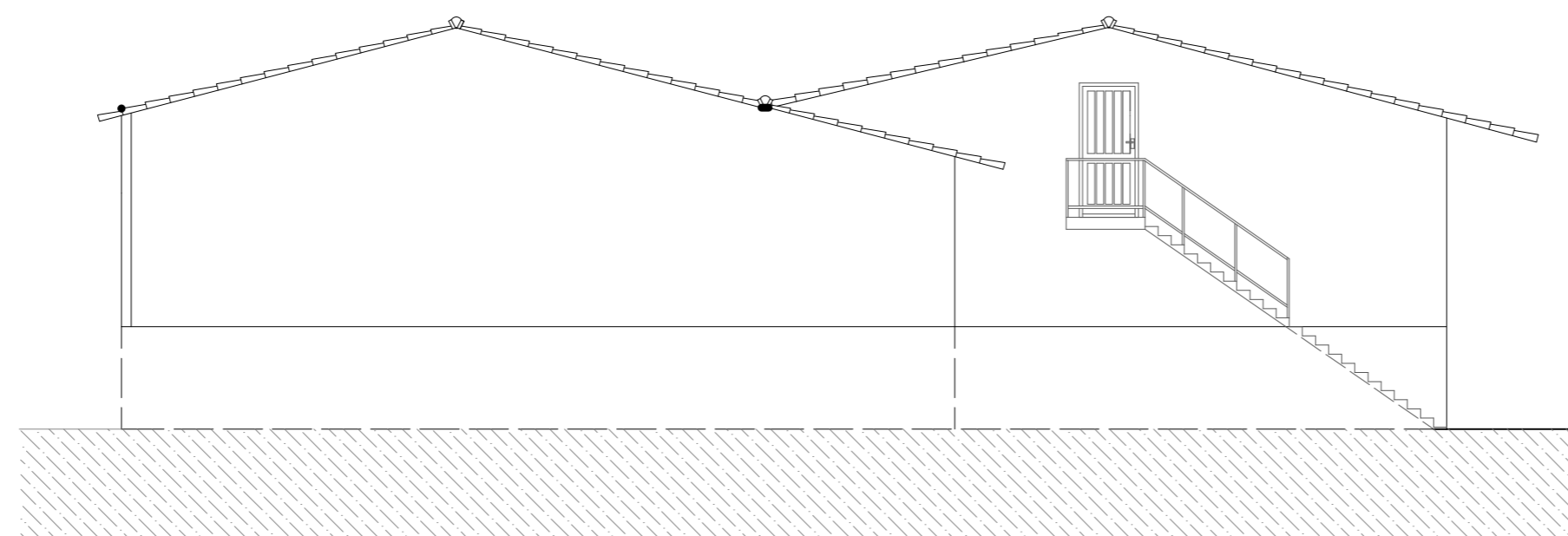
ALÇADO POSTERIOR
