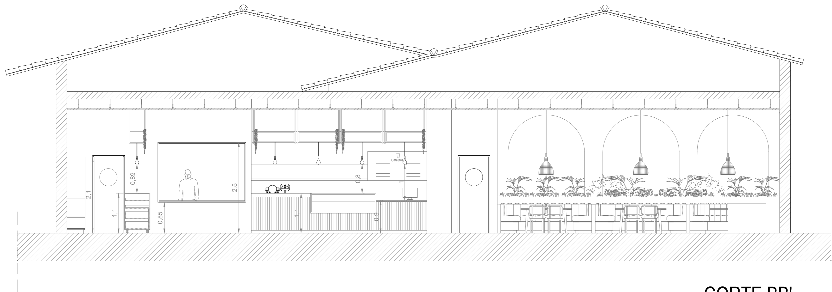
CORTE BB'
