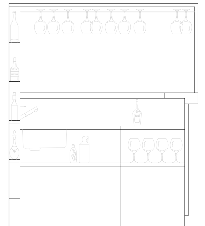
Corte DD'
