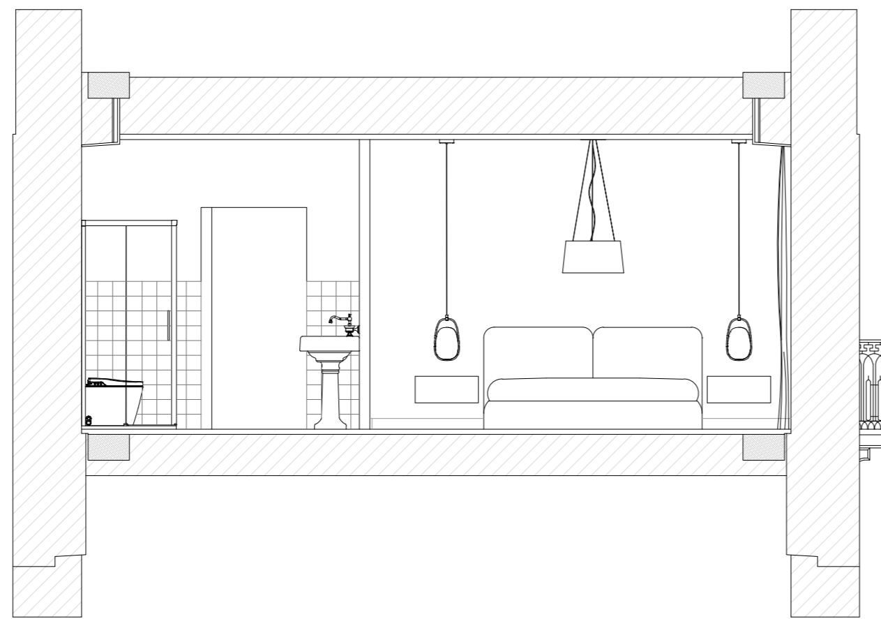
Corte CC'
