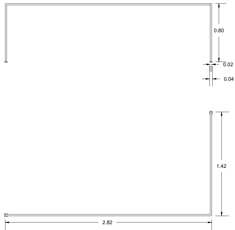
Varão 2
