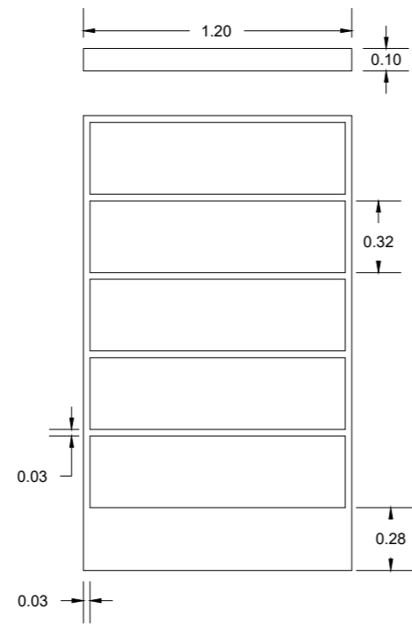
Estante x2
