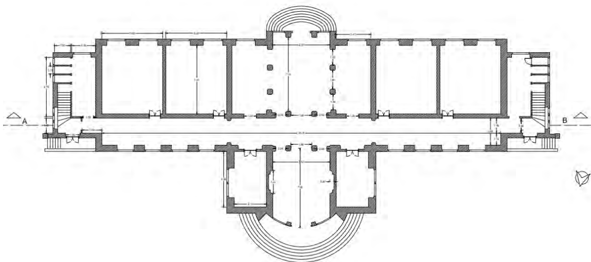
Figura 67 - Planta do Existente Fonte:2023, Maria Luís Martins
