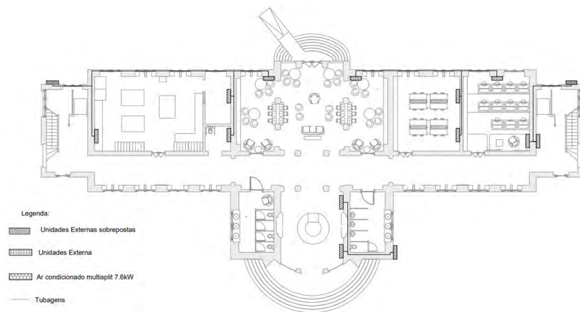
Figura 79 - Planta de Conforto Térmico Fonte: 2023, Maria Luís Martins
