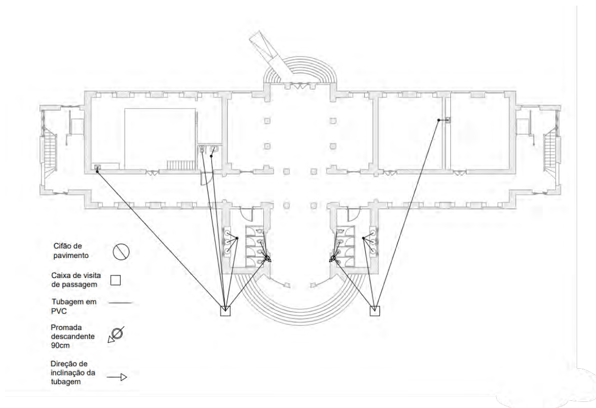
Figura 78 - Planta de Esgotos Fonte: 2023, Maria Luís Martins
