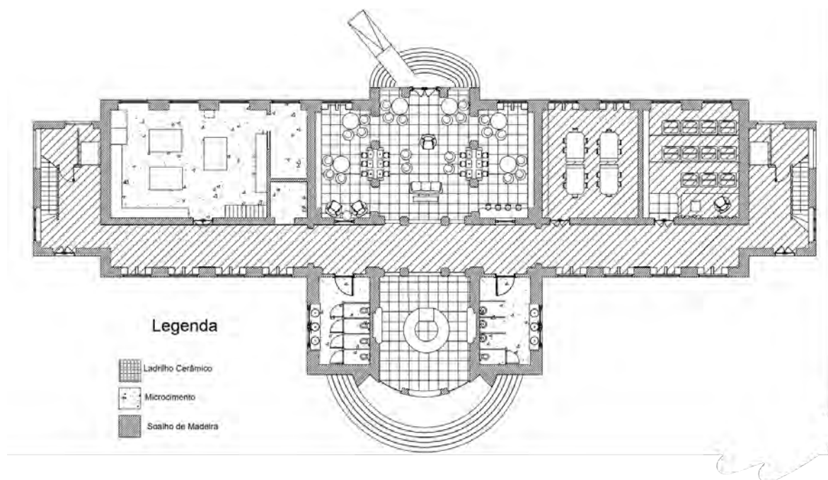
Figura 30 – Planta de Apresentação Fonte: 2023, Maria Luís Martins
