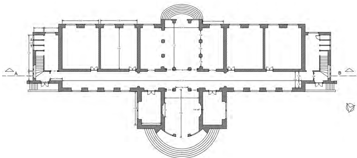
Figura 25 - Planta Original Fonte: 2023, Maria Luís Martins
