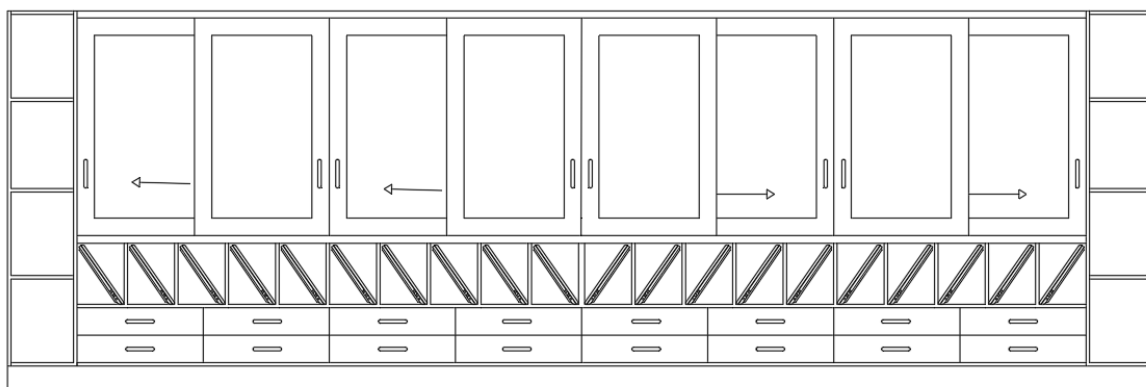
Figura 45 - Projeção do armário Fonte: Maria Luís Martins
