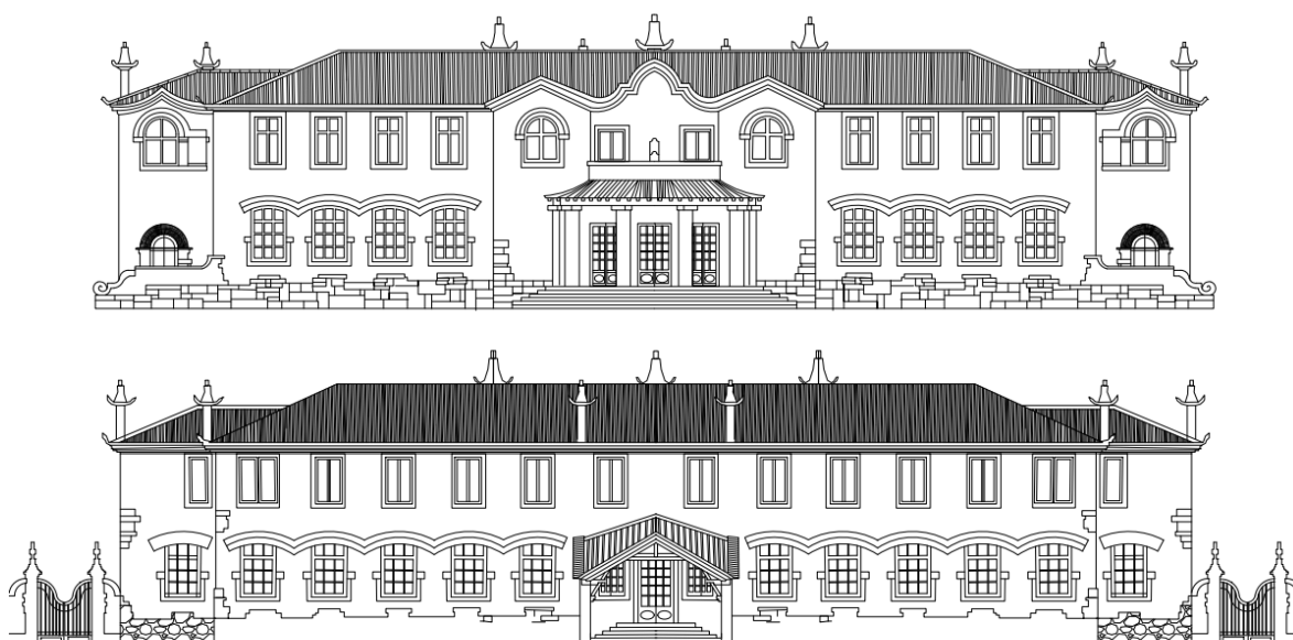
Figura 68 -Alçados Principal e Posterior Fonte: 2023 Maria Luís Martins
