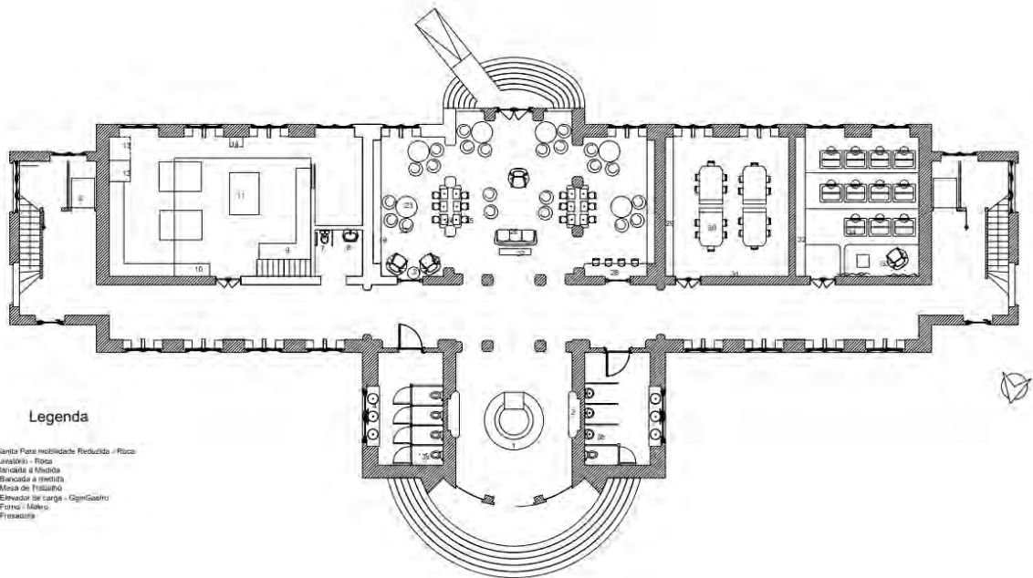
Figura 73 - Planta de Mobiliário e Equipamento, Materiais da Oficina do piso 0 Fonte: 2023, Maria Luís Martins
