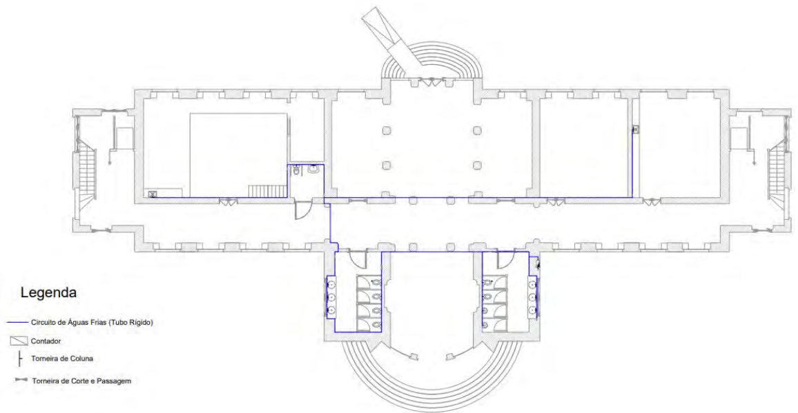
Figura 77 - Planta de Rede de águas Fonte: 2023, Maria Luís Martins
