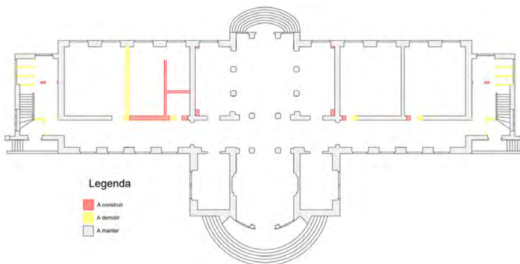
Figura 29 - Planta de Amarelos e Vermelhos. Fonte: 2023, Maria Luís Martins
