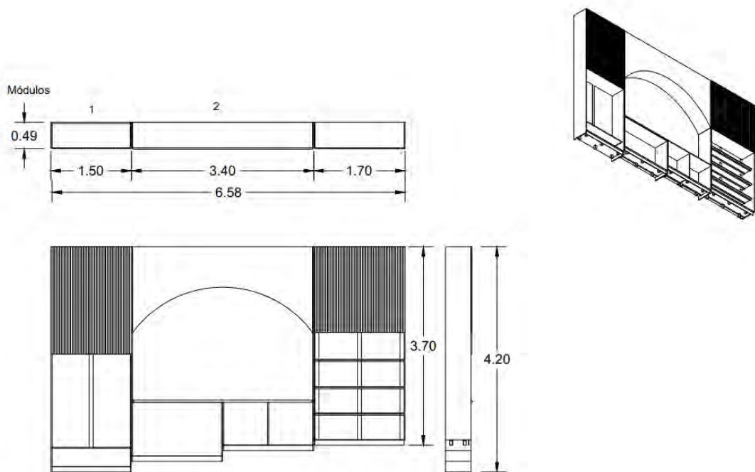
Figura 80 - Desenho de Conjunto Fonte: 2023, Maria Luís Martins
