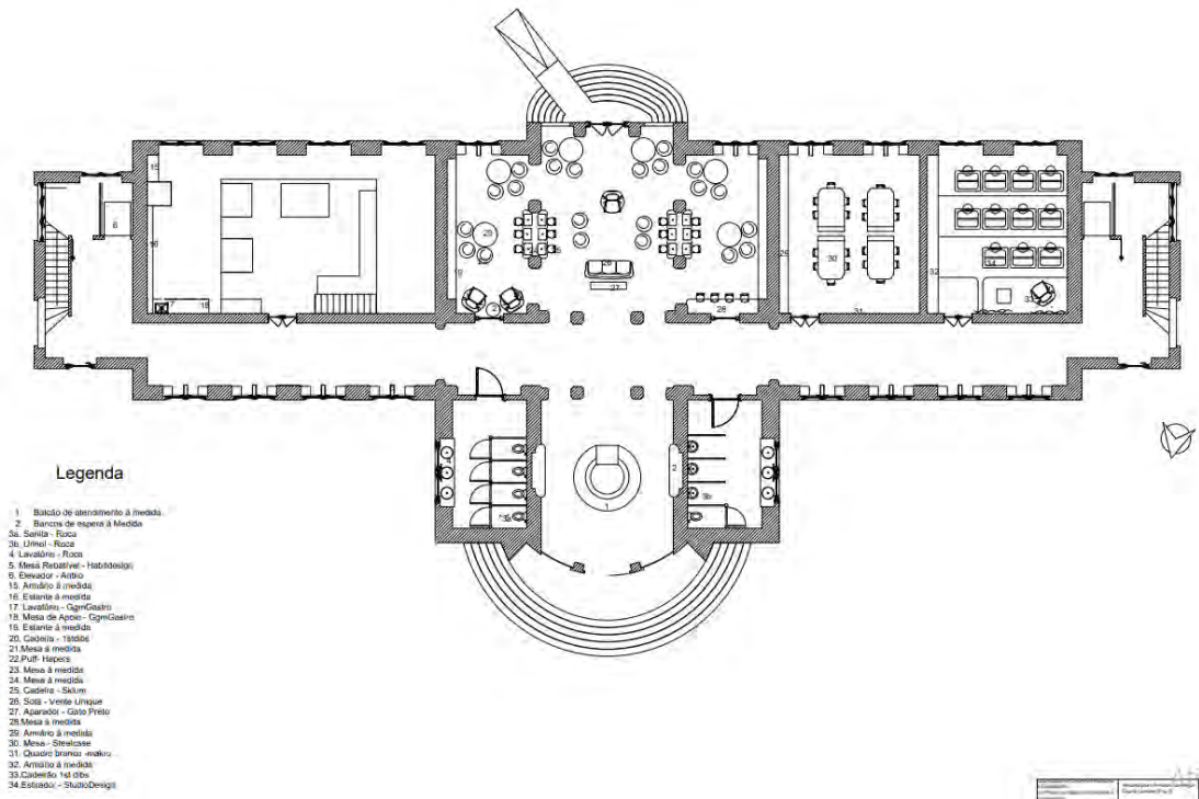
Figura 72 - Planta de Mobiliário e Equipamento Fonte: 2023, Maria Luís Martins
