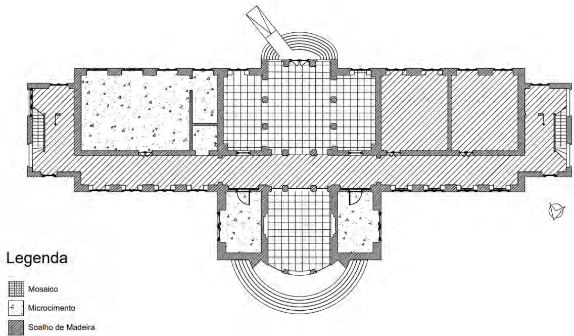
Figura 74 - Planta de Pavimento Fonte: 2023, Maria Luís Martins
