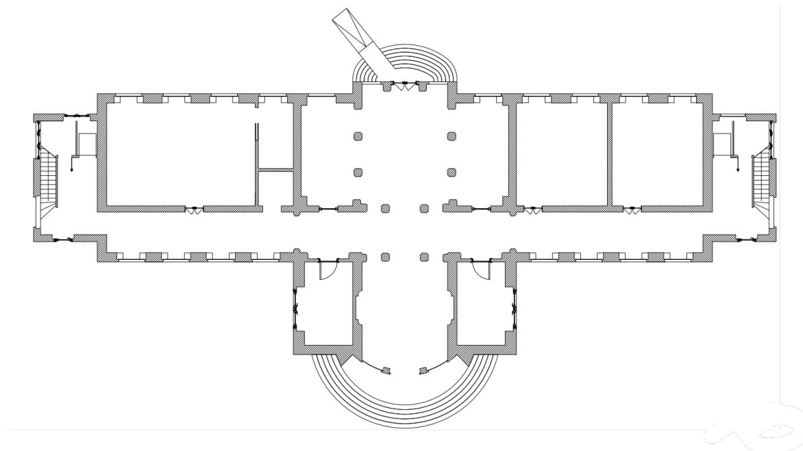
Figura 28 - Planta Final Geral. Fonte:2023, Maria Luís Martins
