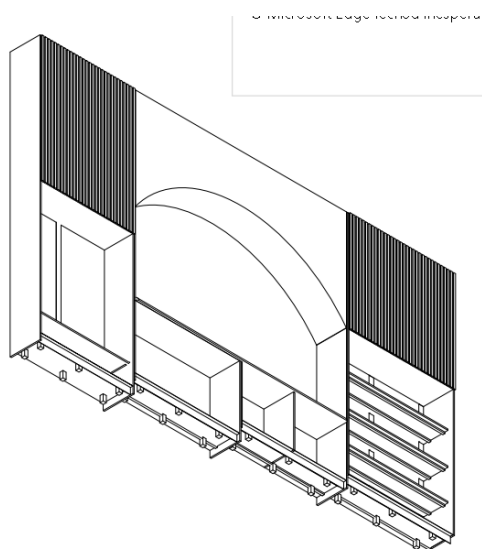
Figura 52 - Axonometria do módulo de arrumação Fonte:2023, Maria Luís Martins
