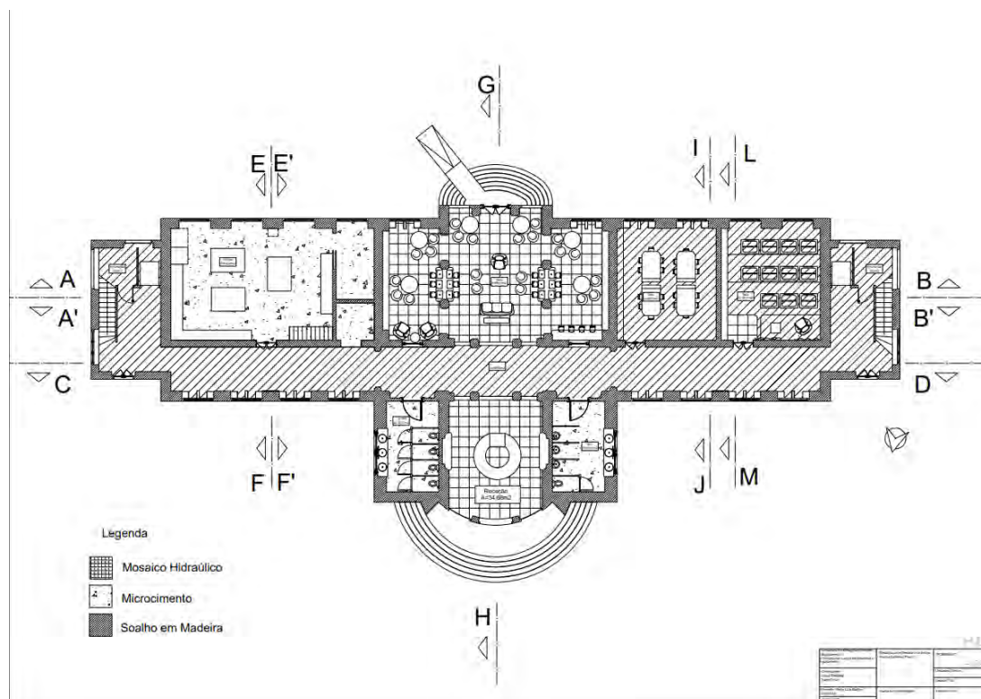
Figura 70 - Planta de Apresentação Fonte: 2023, Maria Luís Martins
