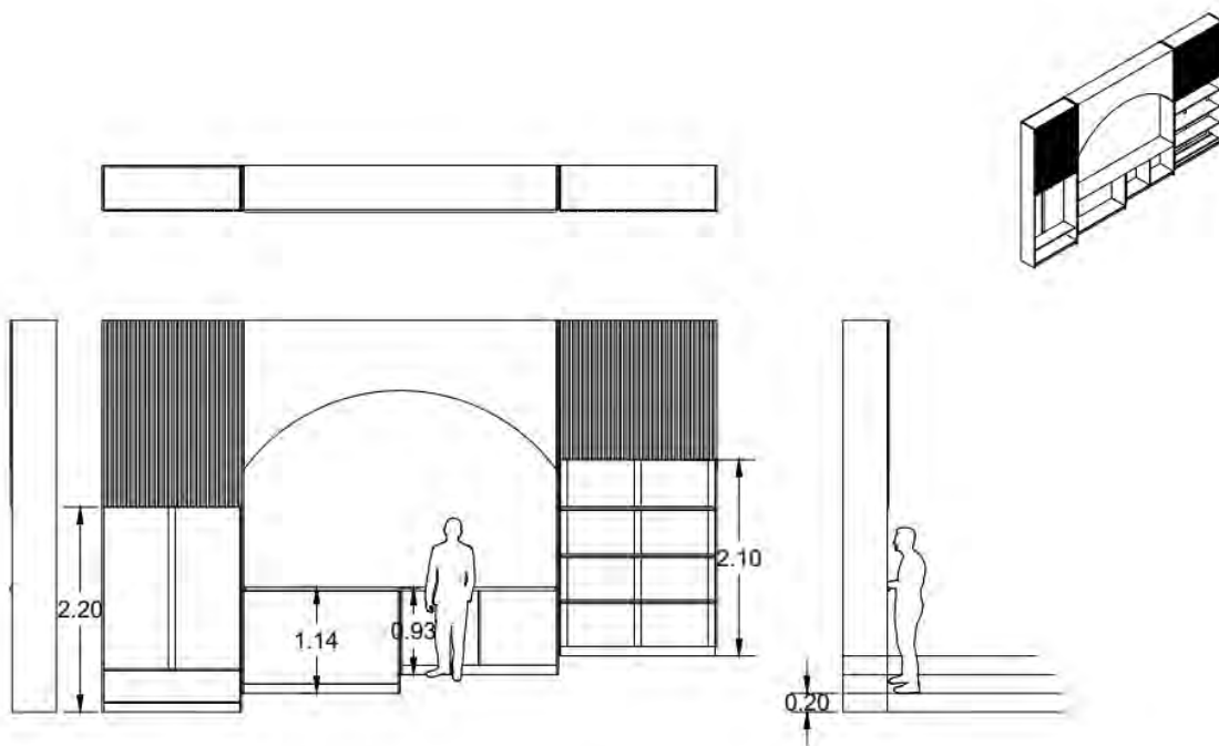
Figura 81 - Desenho de Conjunto com Figura Humana Fonte: Maria Luís Martins
