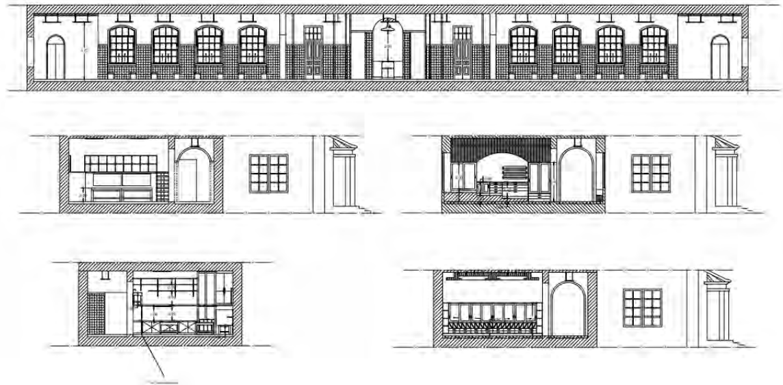
Figura 76 - Cortes CD EF EF', IJ e LM Fonte:2023, Maria Luís Martins
