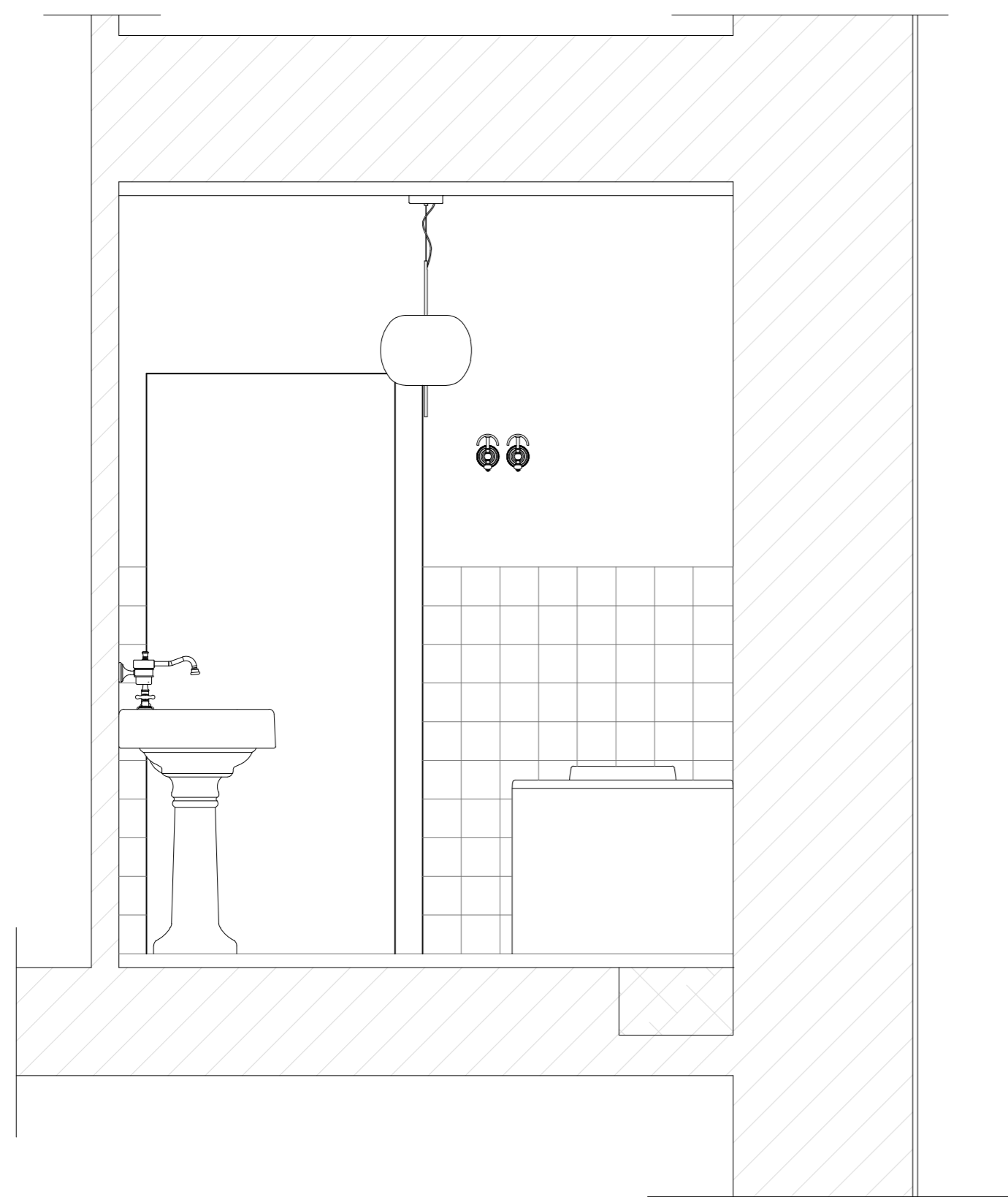
Corte EE'
