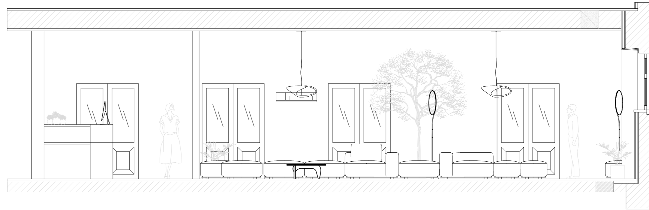
Corte BB'
